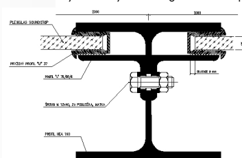
Systém uchycení Plexiglas Soundstop
